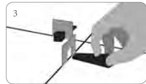
3 COLOCACIÓN DE LAS CUÑAS EN LOS CALZADORES. INSTALLATION OF THE PLASTIC WEDGES INSIDE THE COVER WEDGES. POSE DES CALES EN PLASTIQUE DANS LES CROISILLONS. EINLEGEN DER FLIESENKEILE IN DIE ZUGGLASCHEN.
